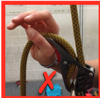
Main de freinage ouverte !
