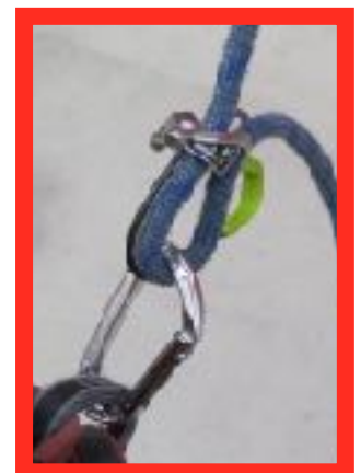
Mousqueton inadapté avec un Mega Jul !
